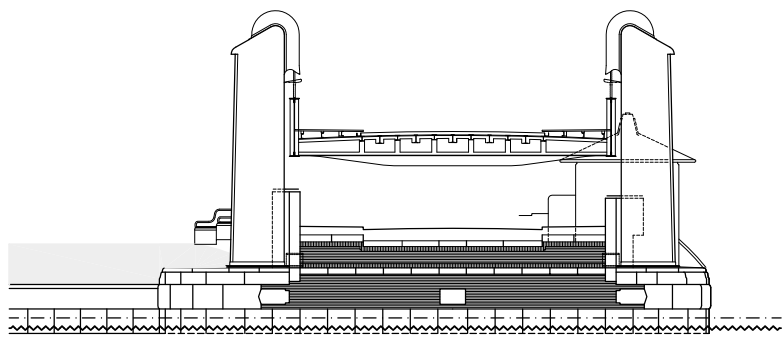
DOORSNEDE AA
