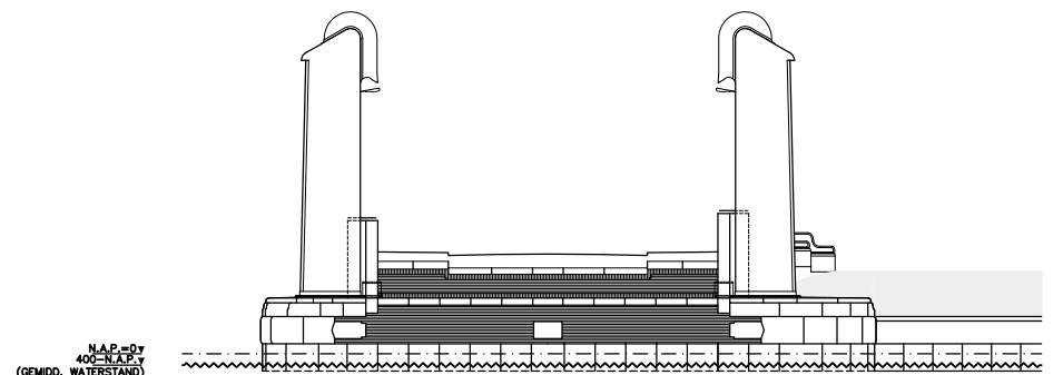
DOORSNEDE BB
