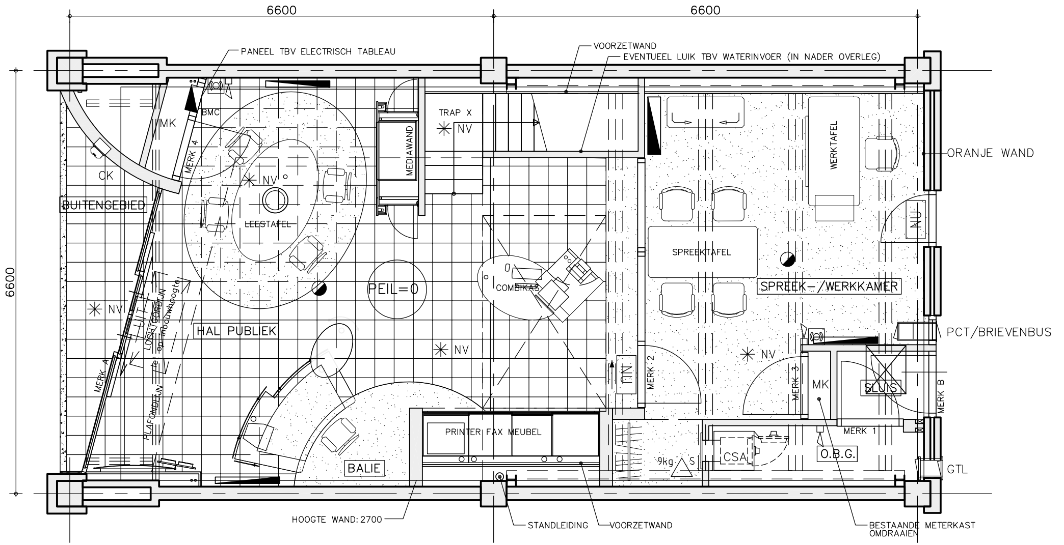
BEGANE GROND
