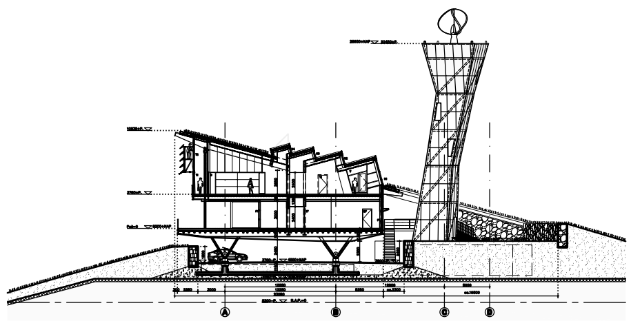
DOORSNEDE B
